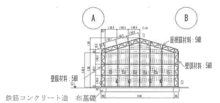
東立面図
