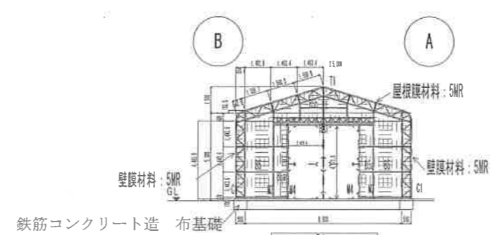
D1 W4000xH4290 西立面図
