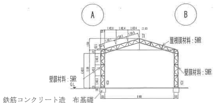
(2)-00 通り軸組図
